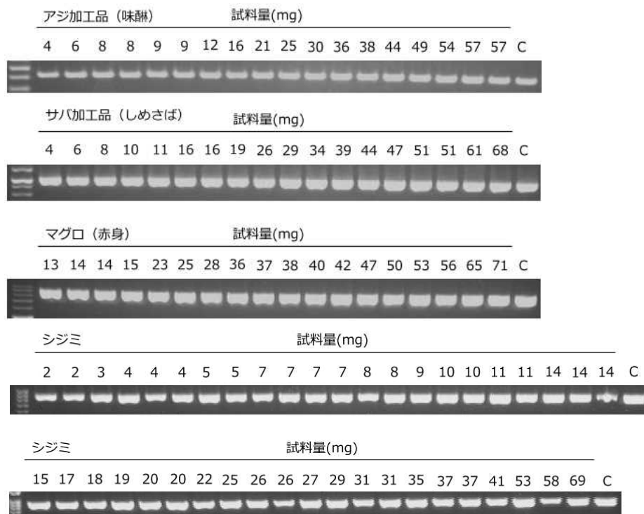
図5 テイル溶解液の添加量を同一にして試料から抽出された DNA の PCR 産物の電気泳動図
