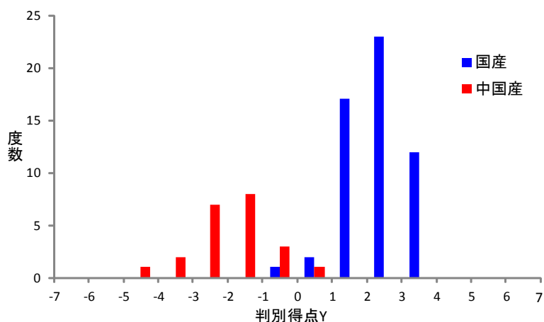
図2 構築した組み合わせ判別モデルの LOOCV 判別得点のヒストグラム
