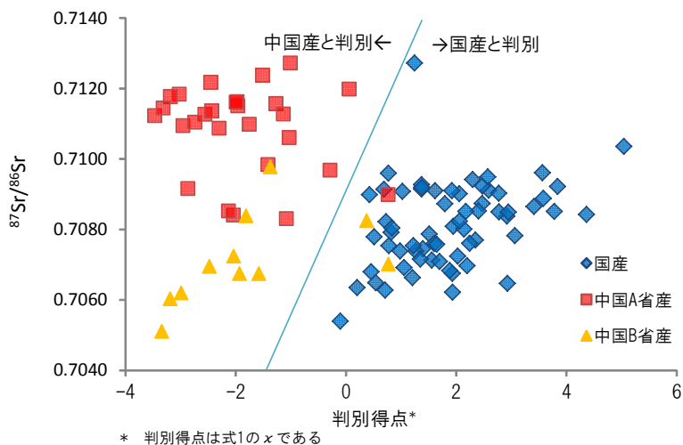
図 5 {}^{87}\text{Sr}/{}^{86}\text{Sr} と元素分析法による判別得点の散布図
