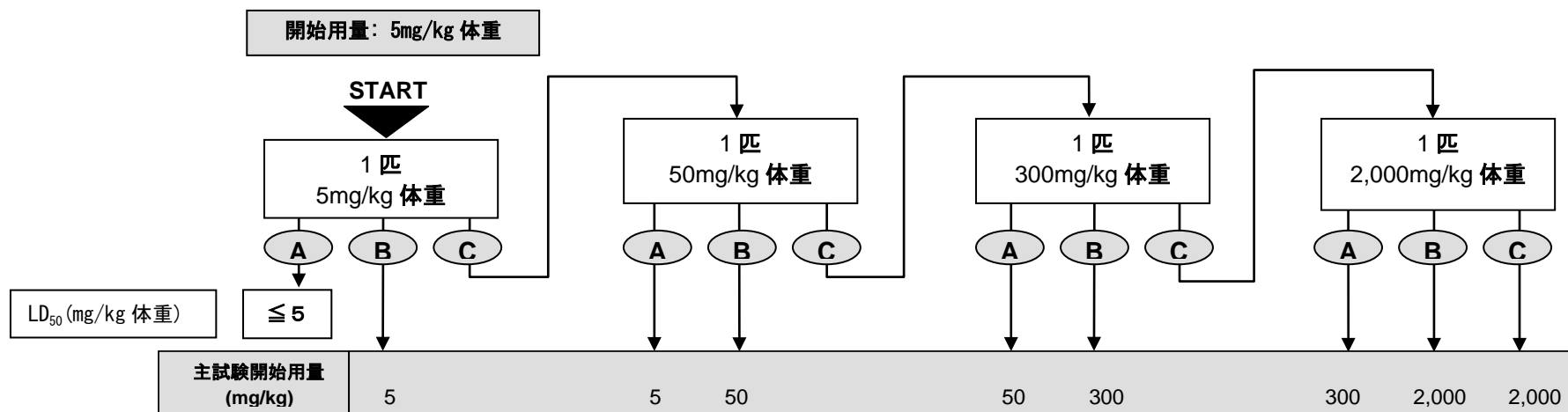
別表 1 : 固定用量法/見当付け試験の手順
